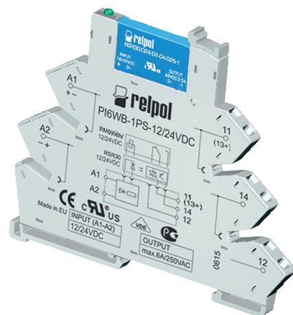
Fot. 2. Przełącznik interfejsowy PIR6WB
