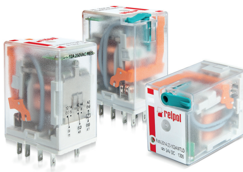
Fot. 4. Nowa linia przekątników R2N, R3N, R4N
